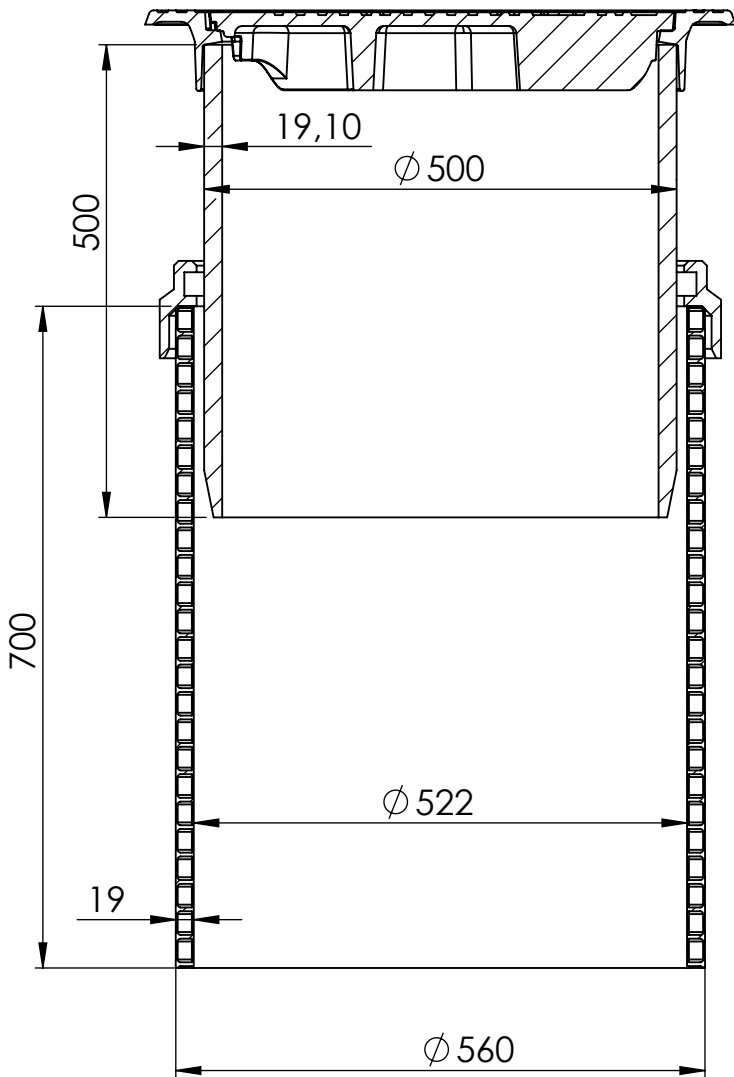
SECTION A-A
