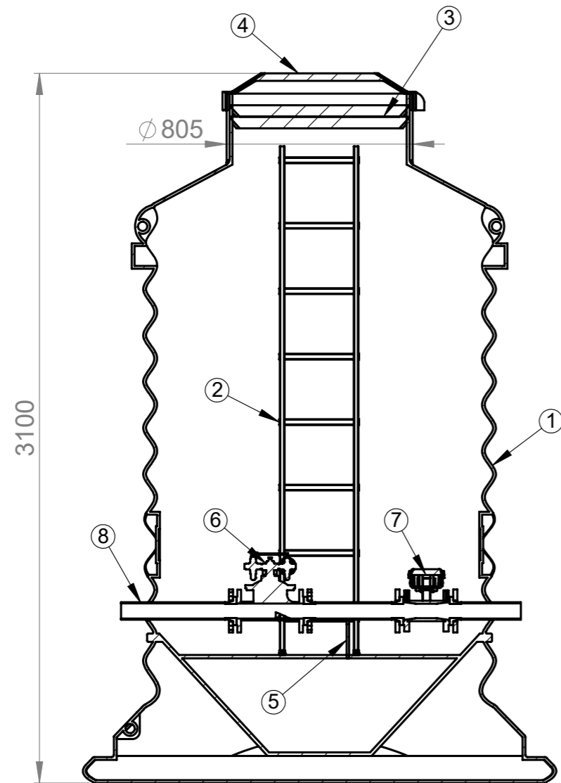
SECTION A-A SCALE 1 : 23
