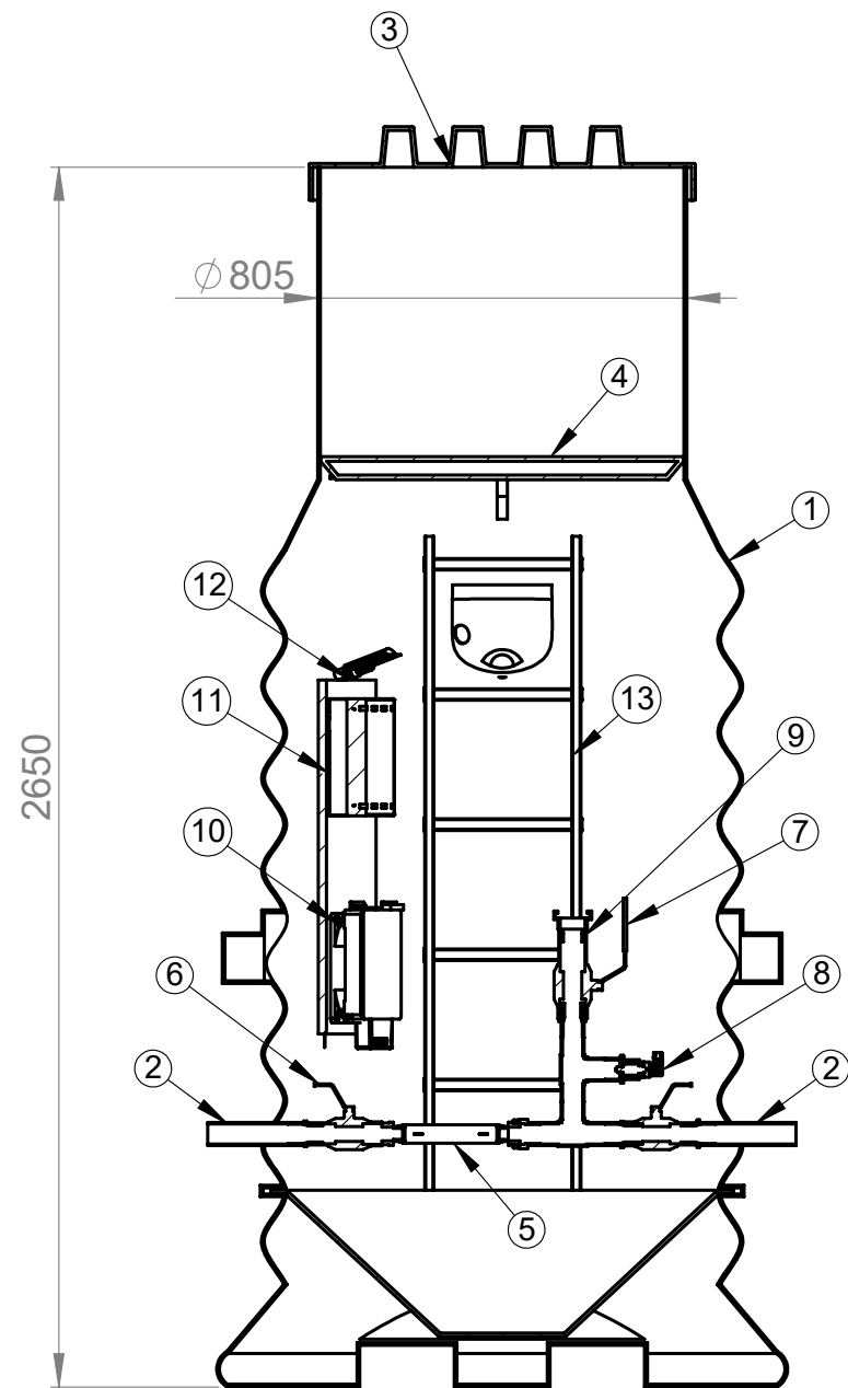
SECTION A-A SCALE 1 : 18
