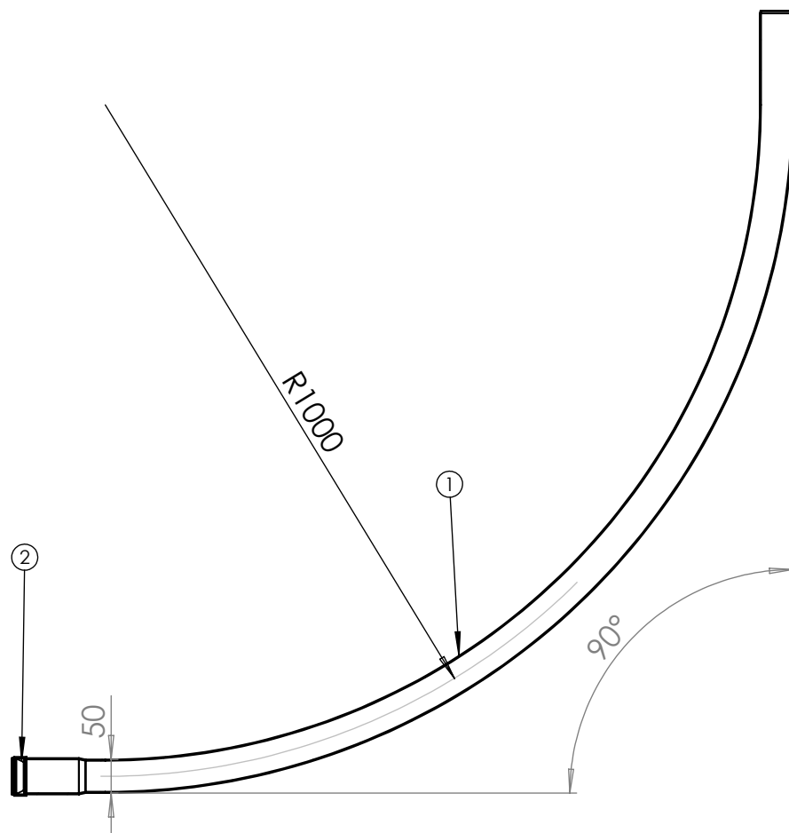
SECTION A-A
