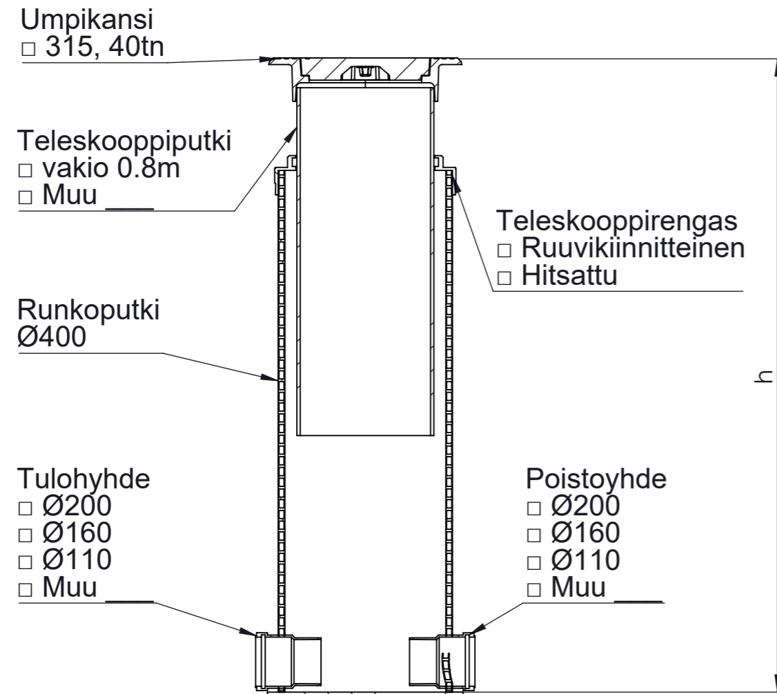
SECTION B-B SCALE 1 : 12
