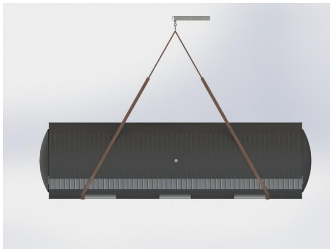
Kuva 1. Vaakamallin noston periaatekuva
